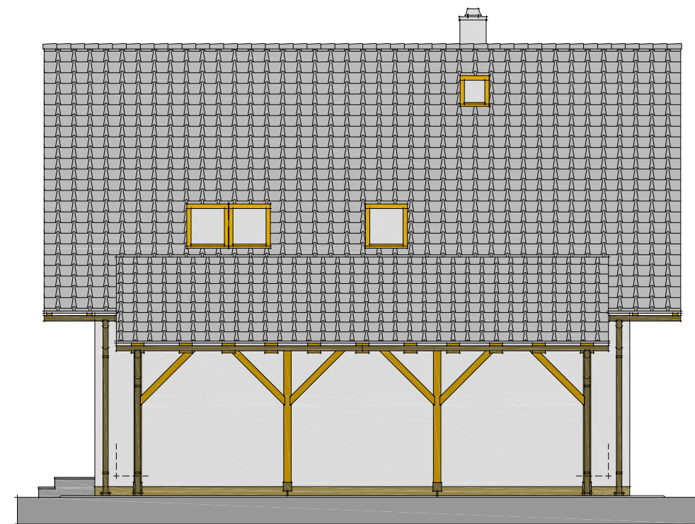
POHLED BOČNÍ
